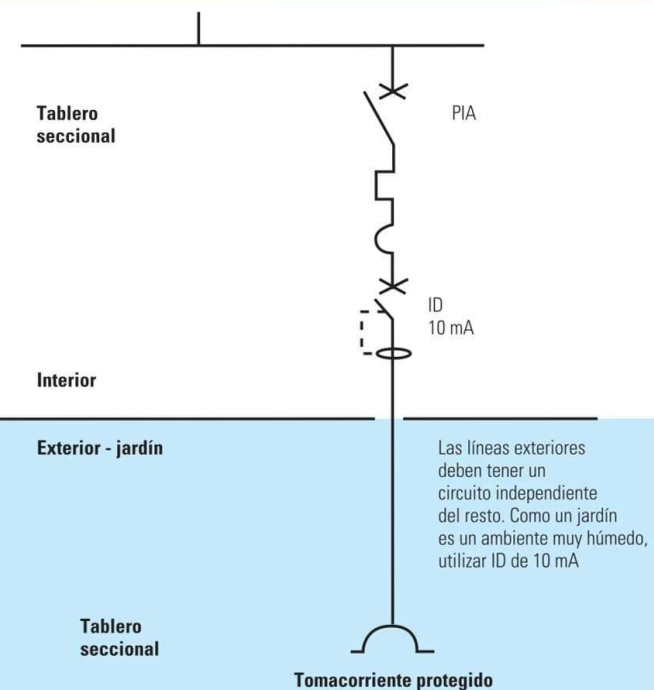
En ambientes húmedos, como un jardín, se debe utilizar el ID de 10 mA. El circuito debe ser independiente para exteriores.
