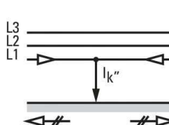
d) Cortocircuito fase-tierra.
