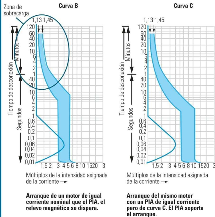
Comparación de las corrientes de sobrecarga para una correcta selección de clase de PIA.
