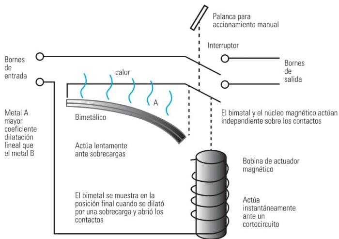
Esquema de funcionamiento de un interruptor termomagnético.
