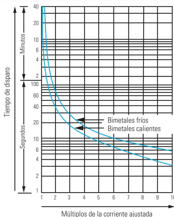
Curvas de respuesta de los relé térmicos, tiempo de actuación en función de veces de la corriente nominal.
