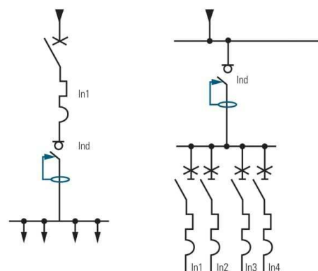
En este caso conviene que la intensidad nominal del ID sea 40% más alta que la del PIA.
