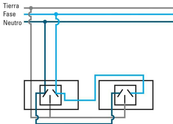
Esquema de conexiones de tomacorrientes.
