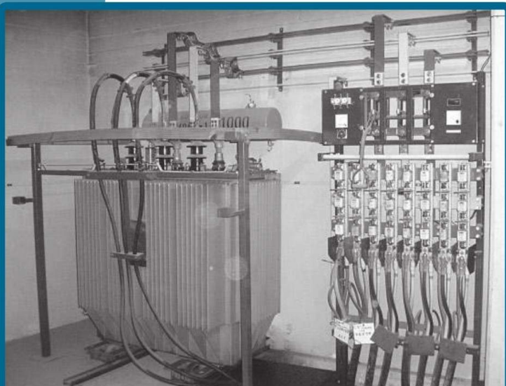
Cámara subterránea de transformación y tablero de distribución a la derecha del transformador, con salida de ocho líneas de distribución en baja tensión.
