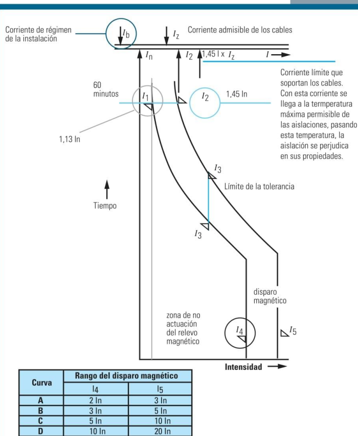
Cómo leer una curva característica y condiciones de selección de PIA para proteger cables.
