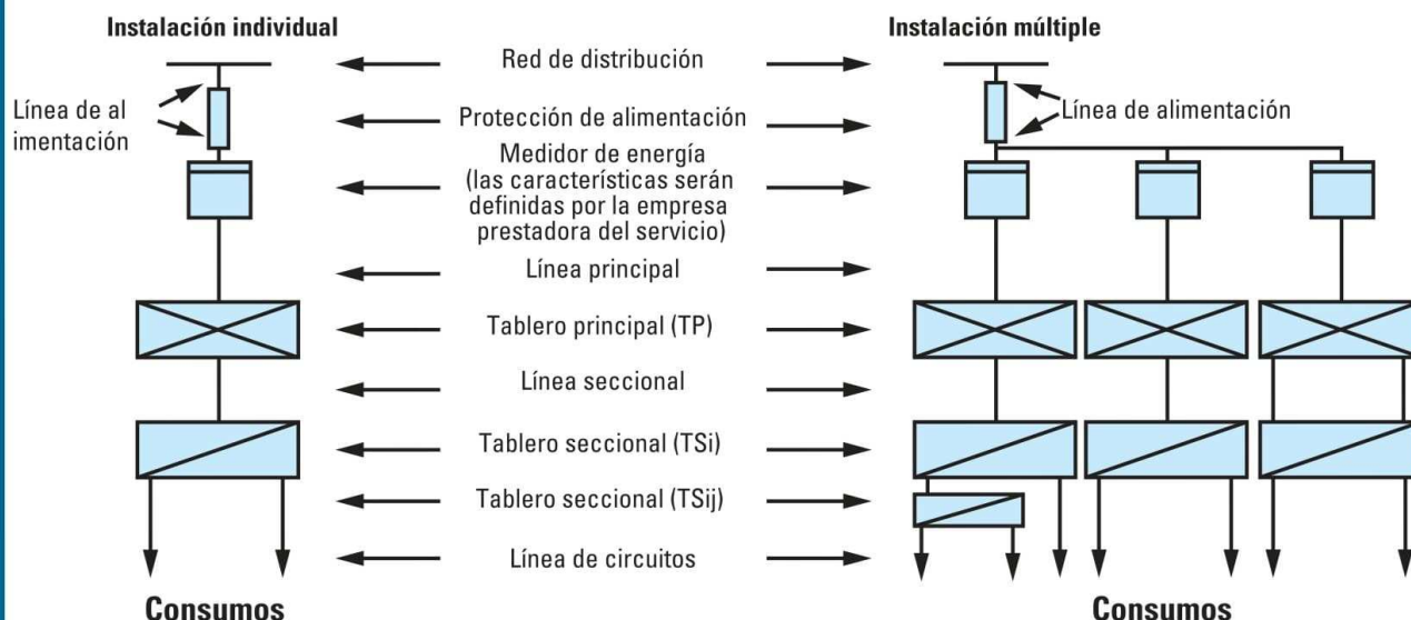
Esquema general de instalaciones que indica las diferentes líneas de baja tensión que estamos analizando.
