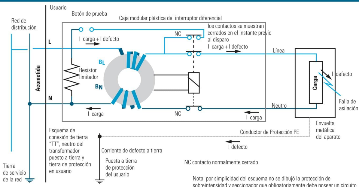
Esquema de funcionamiento de un ID mostrando la necesidad de conductor y puesta a tierra de protección para su funcionamiento.
