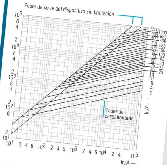
Curva característica y curva de limitación de corriente. Nótese la importancia de la limitación para la protección de la instalación.
