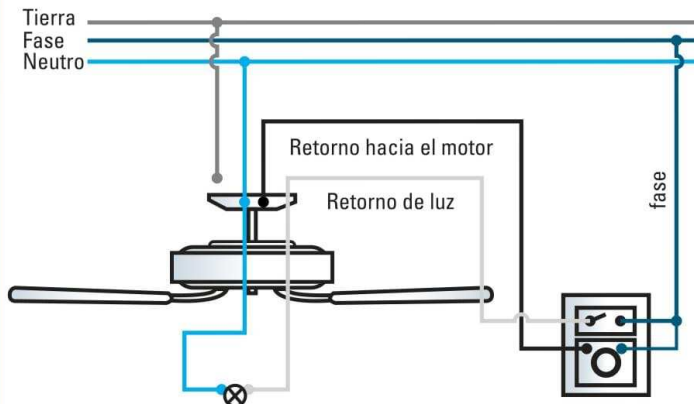
Esquema de conexión de ventilador de techo con artefacto de iluminación.
