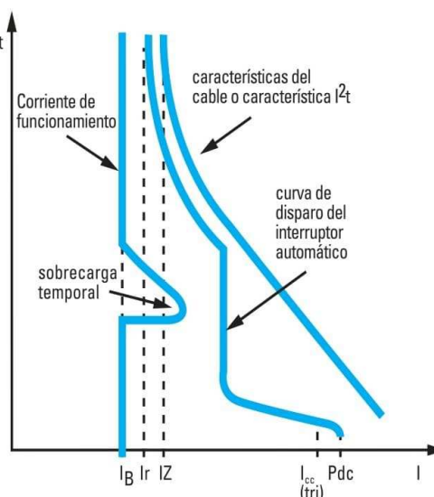
Protección de un circuito por medio de un interruptor automático (termomagnético) PdC: poder de corte.
