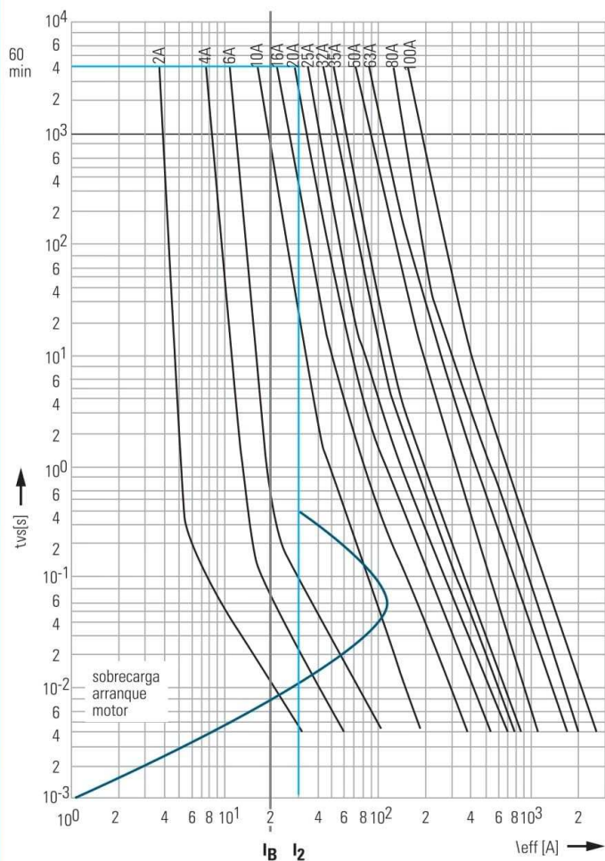
Elección de un fusible usando la curva característica y cumplimiento de las dos condiciones.
