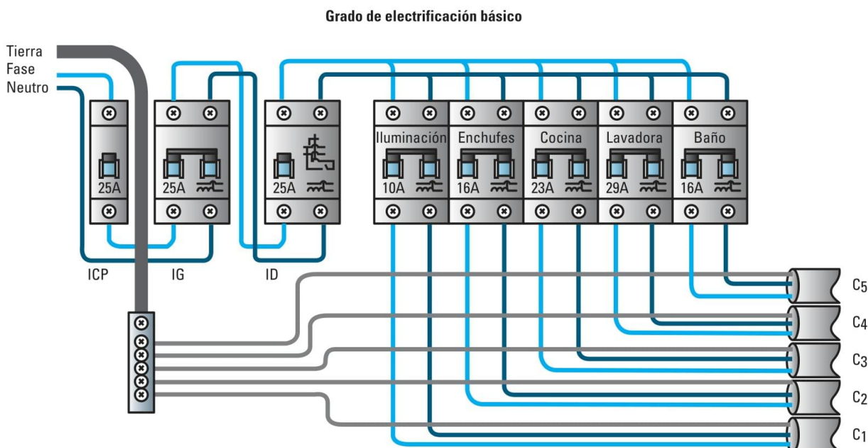
Esquema de cómo deben quedar los circuitos en una instalación eléctrica.
