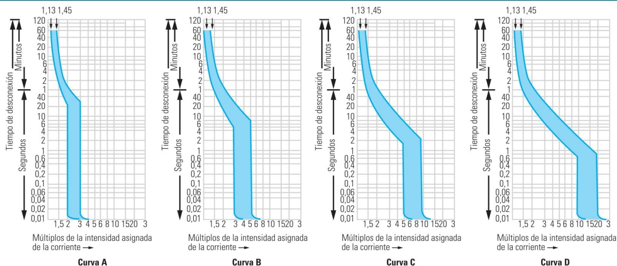
Comparación entre las curvas normalizadas de PIA
