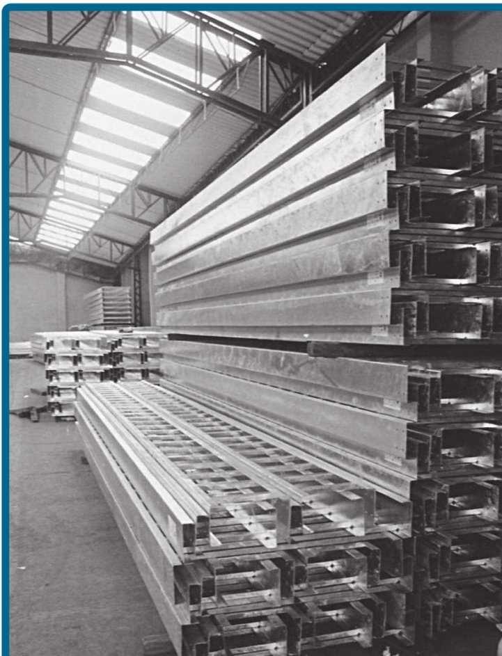
Típicas bandejas perforadas. Las perforaciones preformadas se utilizan para los conectores de unión de las cañerías.
