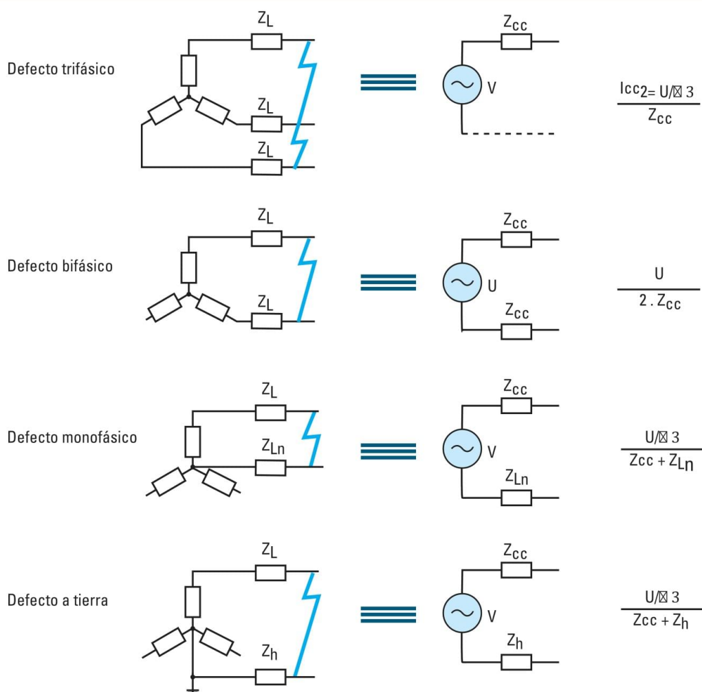
Diferentes corrientes de cortocircuito (trifásico, bifásico, monofásico y contra tierra).
