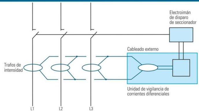
Montaje Nicholson para medir corrientes diferenciales en sistemas trifásicos.
